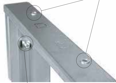
Dado quadro per accoppiamento pannelli (non necessita di chiave) Square nut for panel coupling (no need of wrench)
