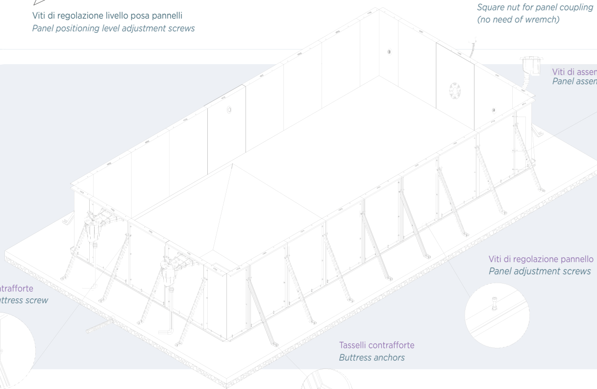
Sistema a incastro senza saldature Snap-on system without welds
